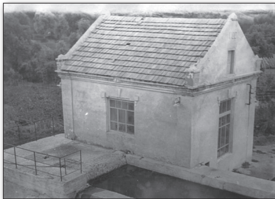
Пуск машинного відділення Політанської ГЕС на р. Мурашка. Фото 7 листопада 1957 р.
